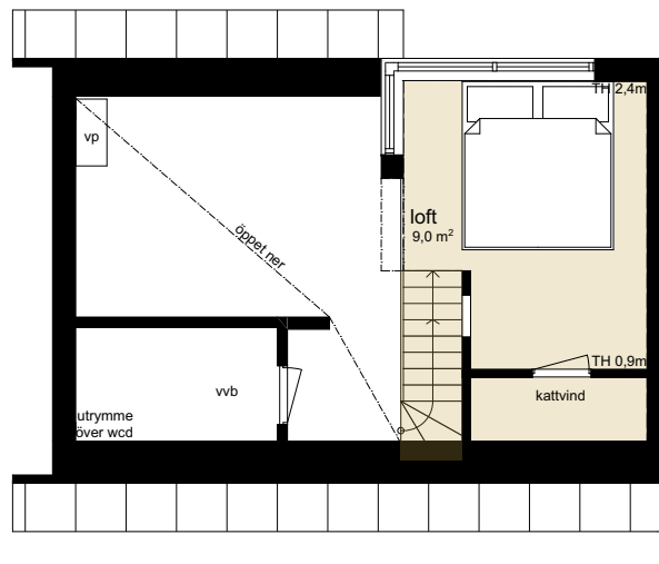
Plan loft
